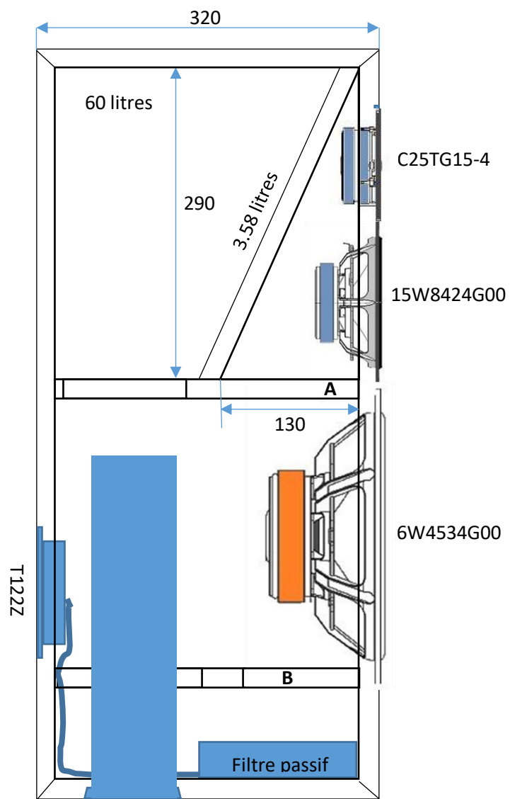
Évent PVC 80x320mm – FC 25Hz
